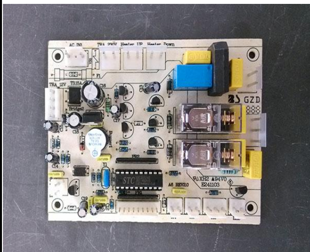
43、主板
