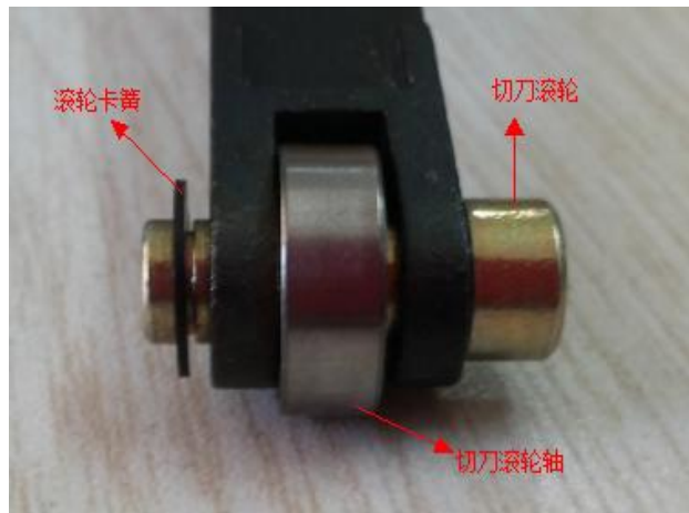
32、切刀滚轮轴/滚轮/滚轮卡簧
